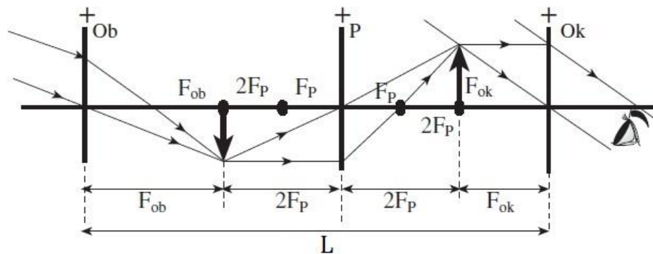
Gambar Pembentukan bayangan pada teropong bumi
